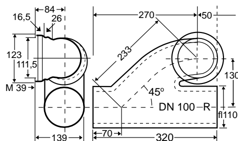
Tegning viser grenrør med høyretilkobling
